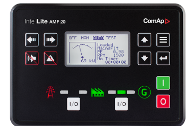
ComAp AMF20
